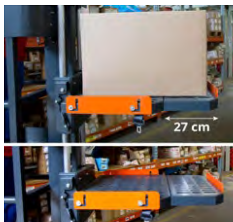
PMF Abnehmbare Erweiterung der Picking-Plattform (für elektrische Kommissionierplattform).
